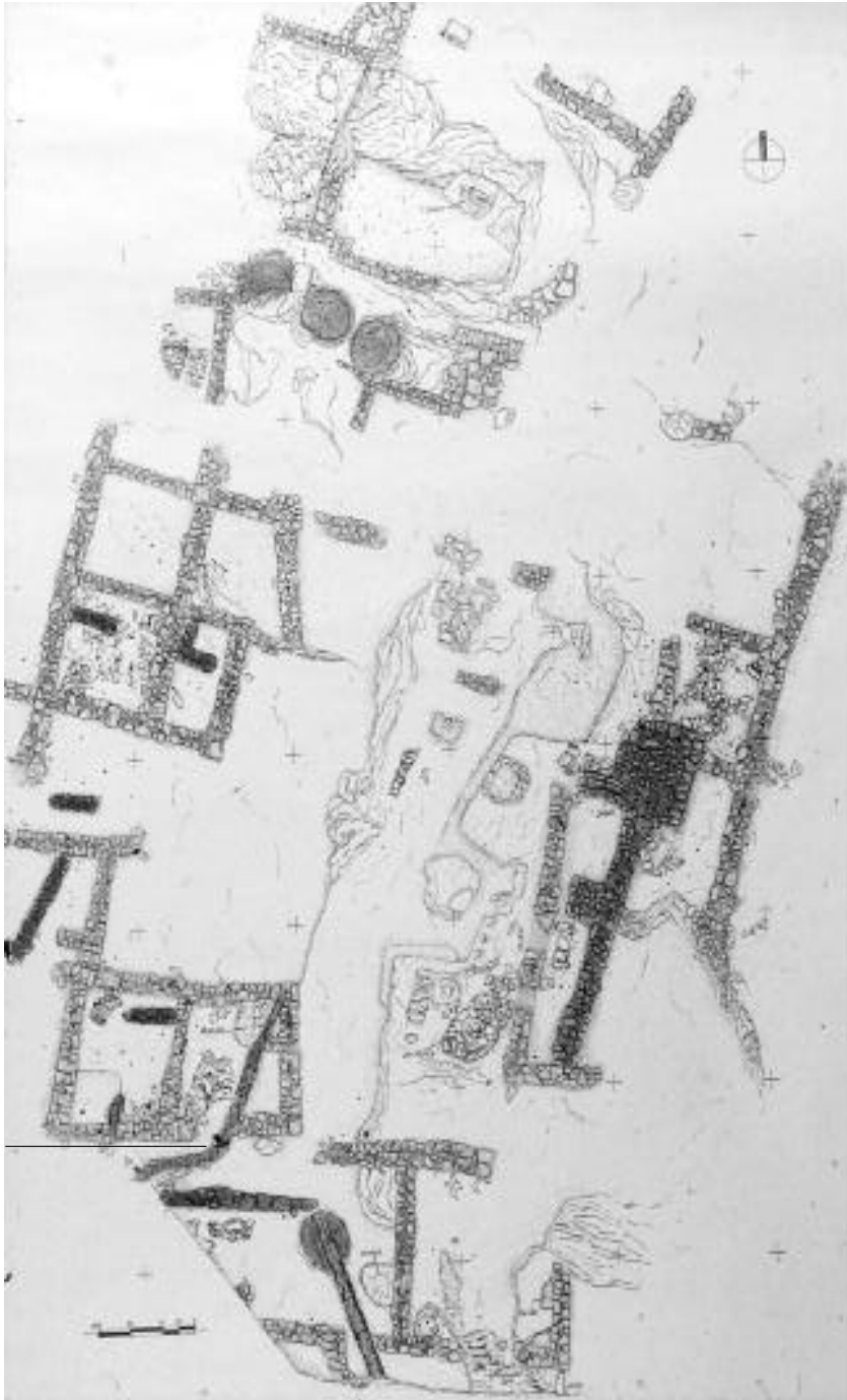
Σχ. 1. Ληγή. Τοπογραφικό σχέδιο τμήματος του οικισμού των ελληγιστικών χρόνων.
