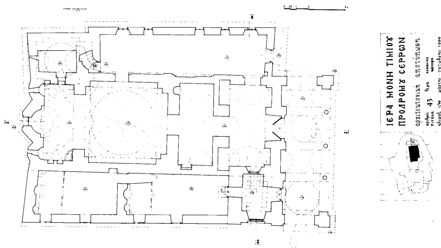
Σχ. 1. Ι. Μ. Τιμίον Προδρομόν Σερρών. Μακρυναγίκι. Κάτοψη.
