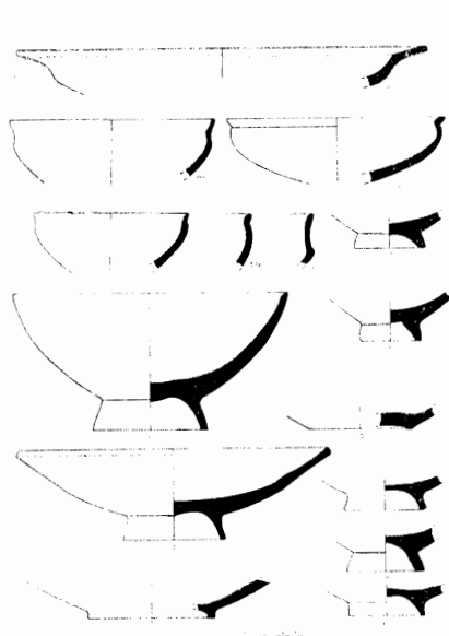
Σχ. 5. Τομές αγγείων
