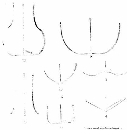
Σχ. 9. Τομές γυάλινων αγγείων
