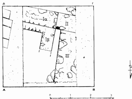
Σχ. 3. Τομή Α/1983. Κάτοψη
