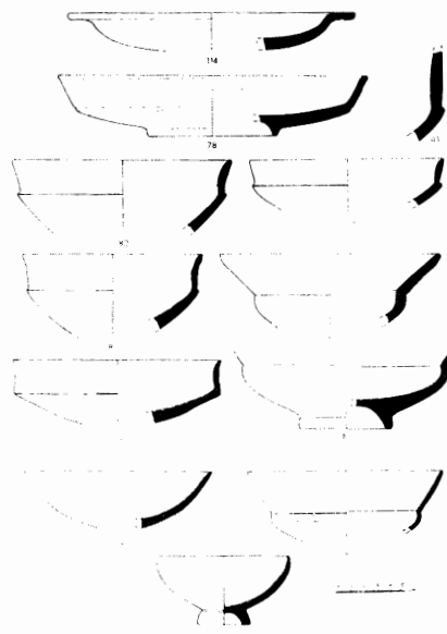
Σχ. 6. Τομές αγγείων
