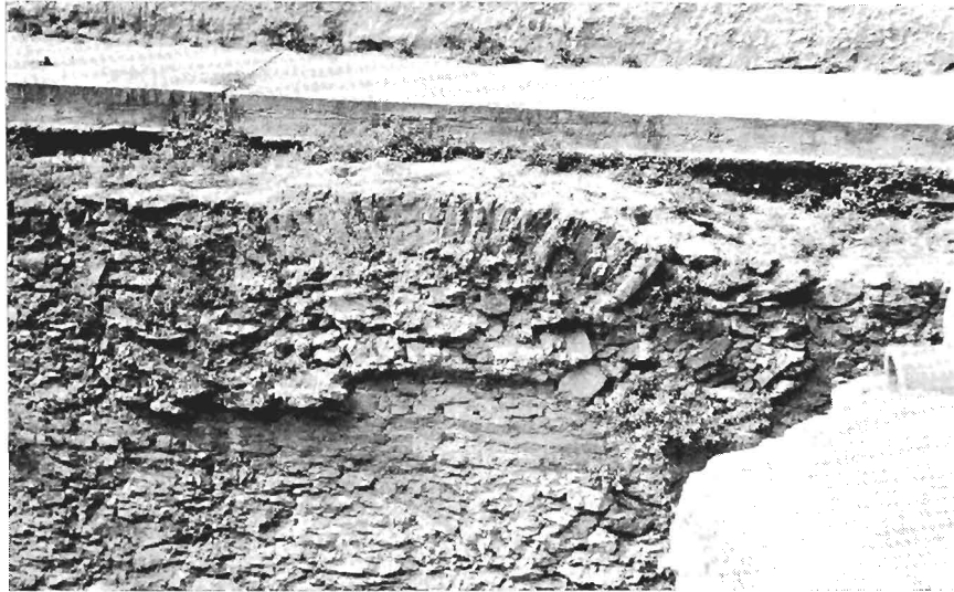
α. Τὸ ἀνακουφιστικὸ τόξο στὸ νότιο στυλοβάτη τοῦ κεντρικοῦ κλίτους τοῦ ναοῦ Α.
