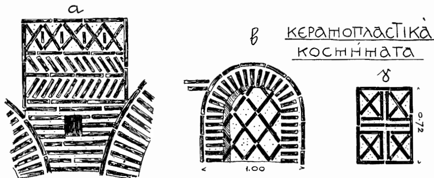
Εἰκ. 5. Λεπτομέρειαι τῶν κεραμοπλαστικῶν κοσμημάτων τῆς κινστέρας
