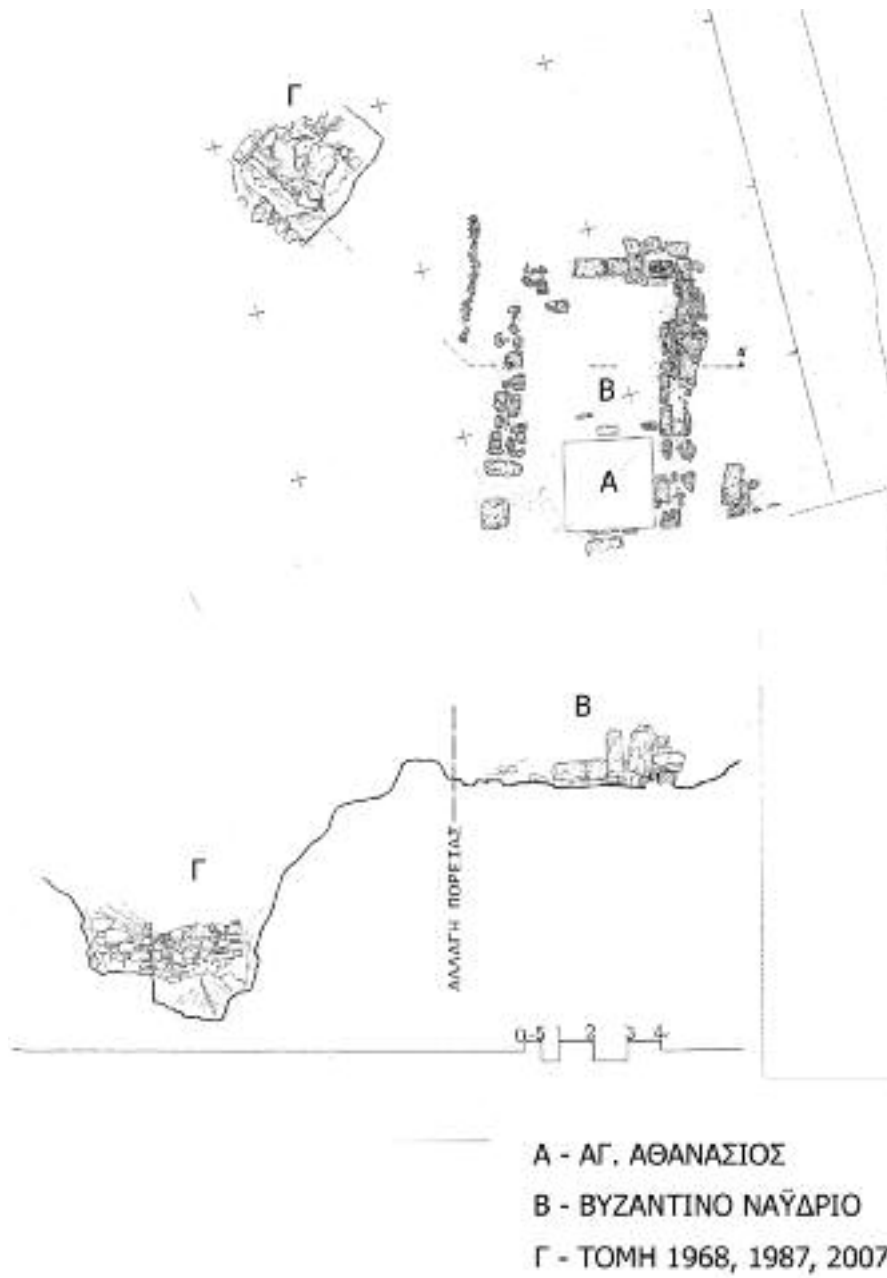
Εικ. 3. Σχεδιαστική αποτύπωση ανασκαφής Αγίου Αθανασίου κατά το 2007.
