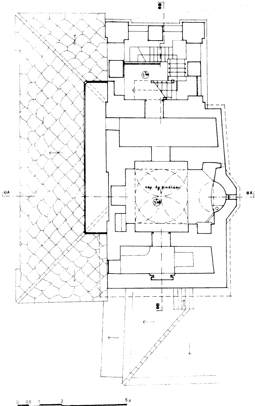
Σχ. 3. Ι. Μ. Τιμίον Προδροίμου Σεργίων. Παρεκκλήσιο Αγίου Νικολάου. Κάτοψη (αρχιτέκτων Π. Ξύδας).
