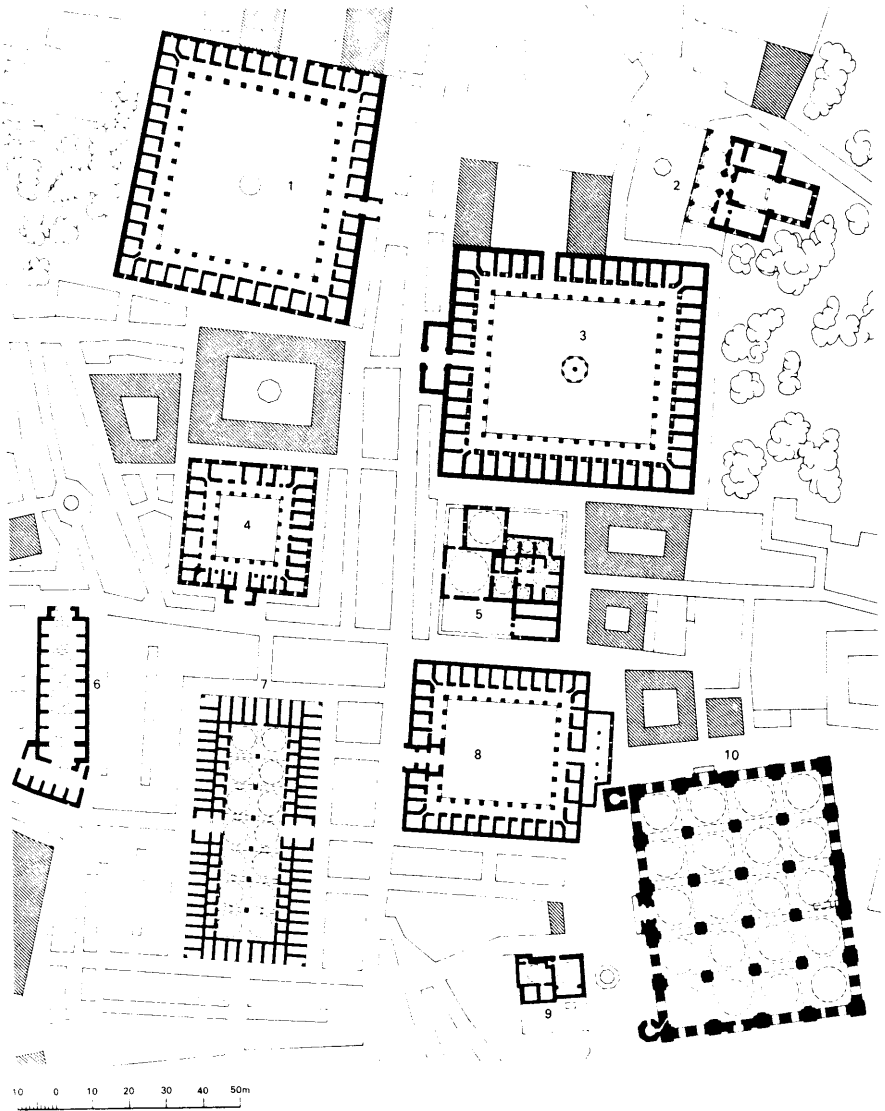
Σχ. 2. Κάτοψη του μπεζεστενίου της Προύσας και του Ulu camii (7 μπεζεστένι - 10 Ulu camii) (από το αρχείο της 9ης Εφορείας Βυζ. Αρχαιοτήτων - της Π. Αστροεινίδου - σχεδ. παρουσίαση Ε. Μάλλη).
