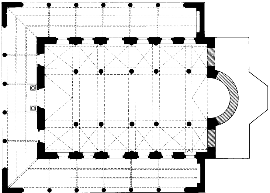
Εικ. 16. Κοίμηση Θεοτόκου Ερμούπολης (1828-1829). Κάτοψη ισογείου. Γραφική αποκατάσταση του αρχικού σχεδίου. Πηγή: Ι. Τρανού - Α. Κόκκου, Ερμούπολη, Αθήνα 1980, σ. 89.
