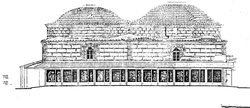
Σχ. 5. Υπόχουσα βόρεια όψη (οδός Βασ. Ηρακλείου).
