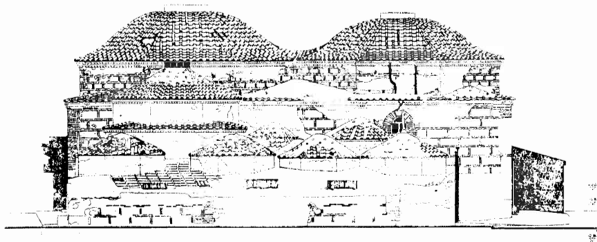
Σχ. 6. Υπόχουσα νότια όψη (οδός Φραγκίνη).
