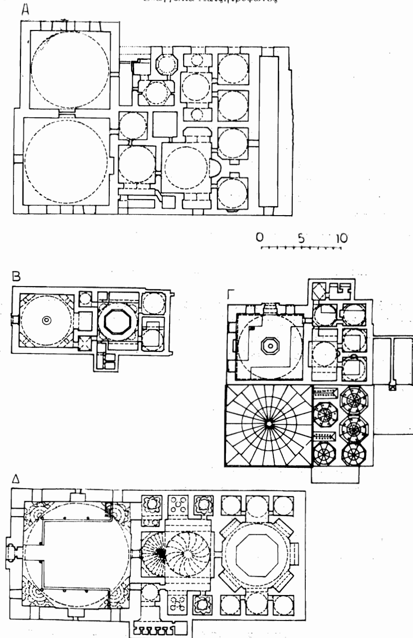
Σχ. 10. Α. Pazar ή Yahudi hammamί στη Θεσσαλονίκη. Β. Cagir hammamί στην Προύσα. Γ. Mustafa Pasa hammamί στο Izmid. Δ. Mahmud Pasa hammamί στην Κωνσταντινούπολη.
