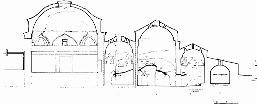
Σχ. 12. Κατά μήκος τομή.
