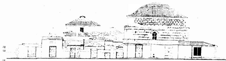
Σχ. 6. Υπόχουσα νότια όψη (οδός Φραγκίνη).
