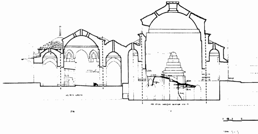
Σχ. 13. Τομή κατά πλάτος των ζεστών χώρων.
