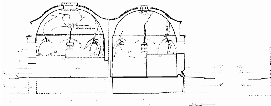
Σχ. 11. Τομή στους μεγάλους τρούλους.
