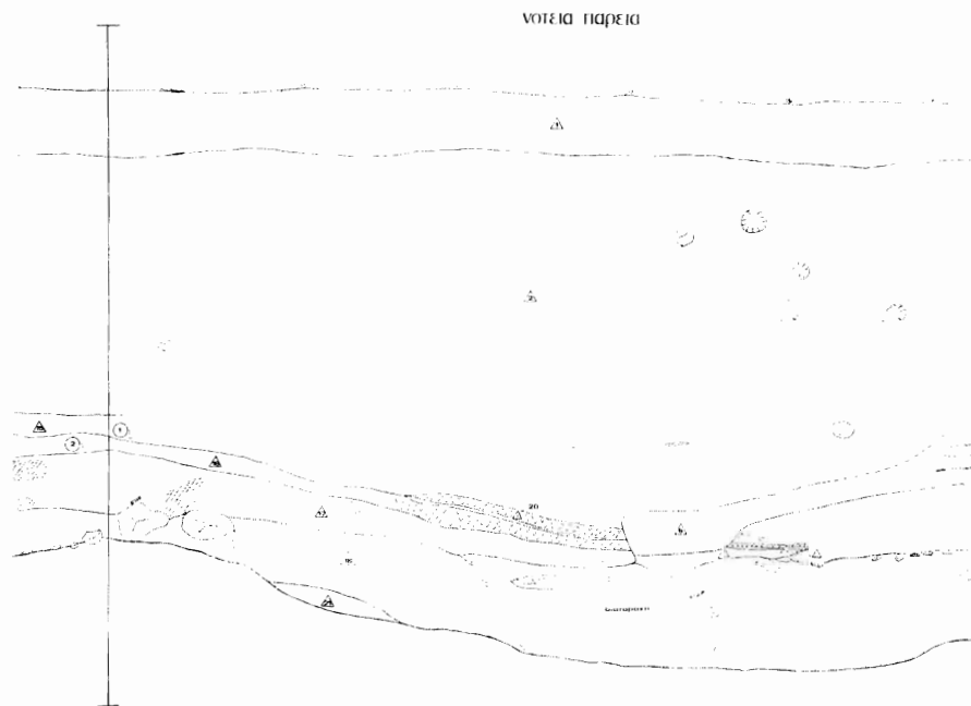
Σχ. 3. Στρωματογραφία
