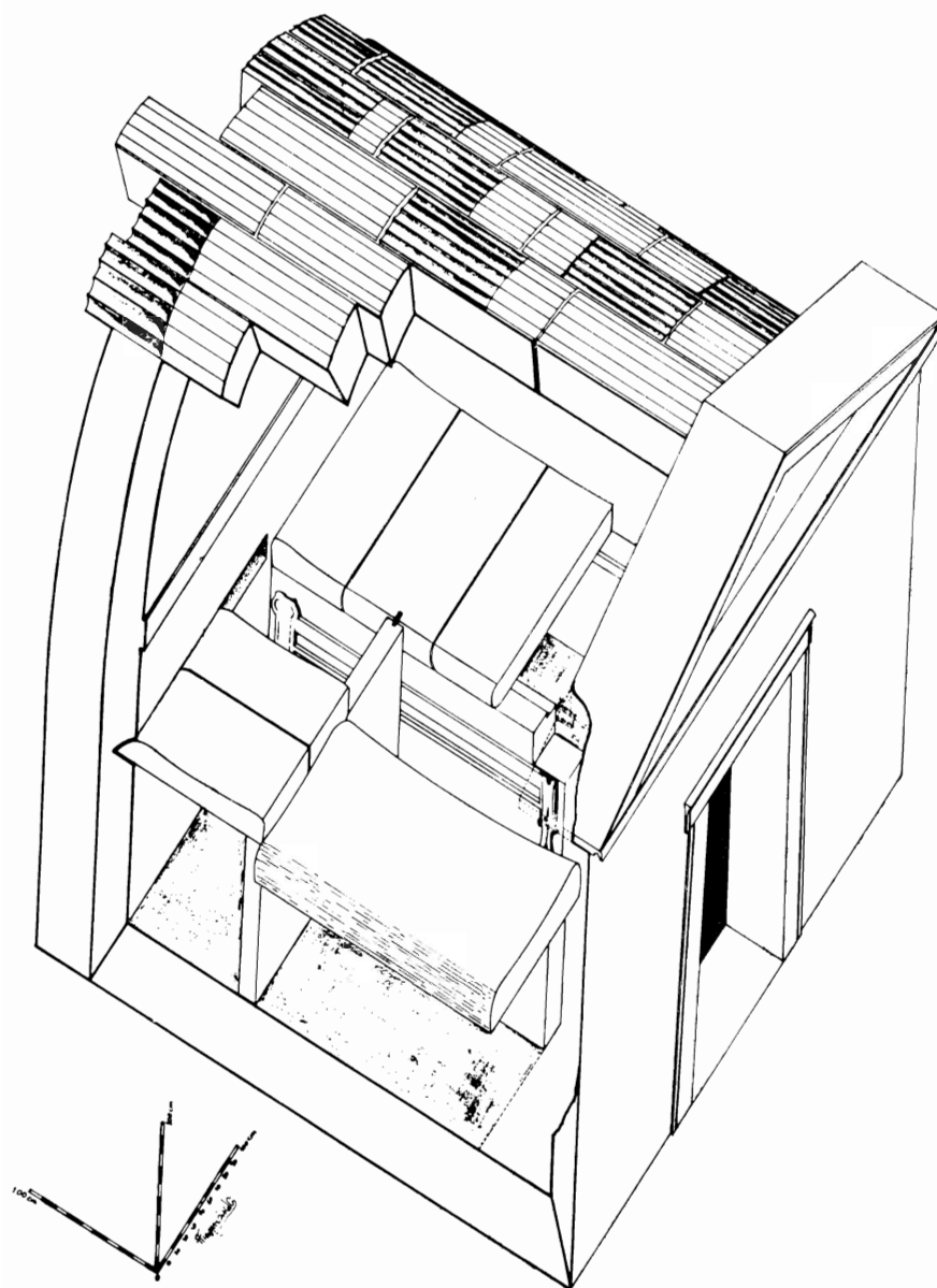
Σχέδ. 2. Αξονομετρικό σχέδιο του τάφου.
