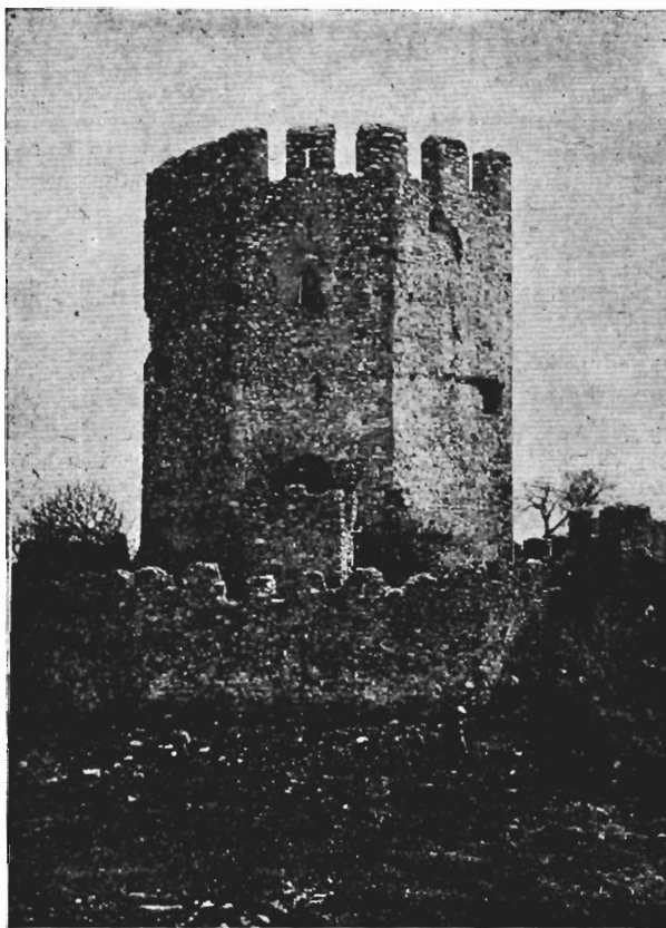
Εἰκ. 9. Νοτιοδυτικὴ ἄποψη τοῦ κεντρικοῦ πύργου. Μπροστὰ του διακρίνεται ἡ τρίτη γραμμὴ τοῦ τείχους καὶ τὸ προτείχισμα, πὸν υπερασπίζει τὴν εἴσοδο τοῦ πύργου.
